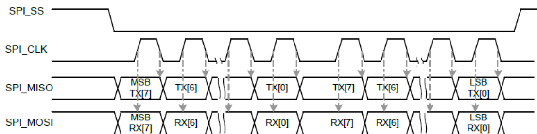
圖 1.1 SPI 時序圖
